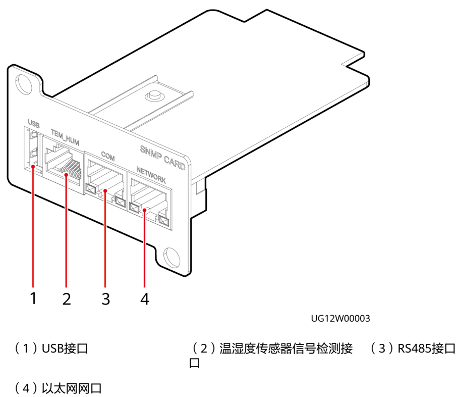
图 4-5 SNMP 卡外观
