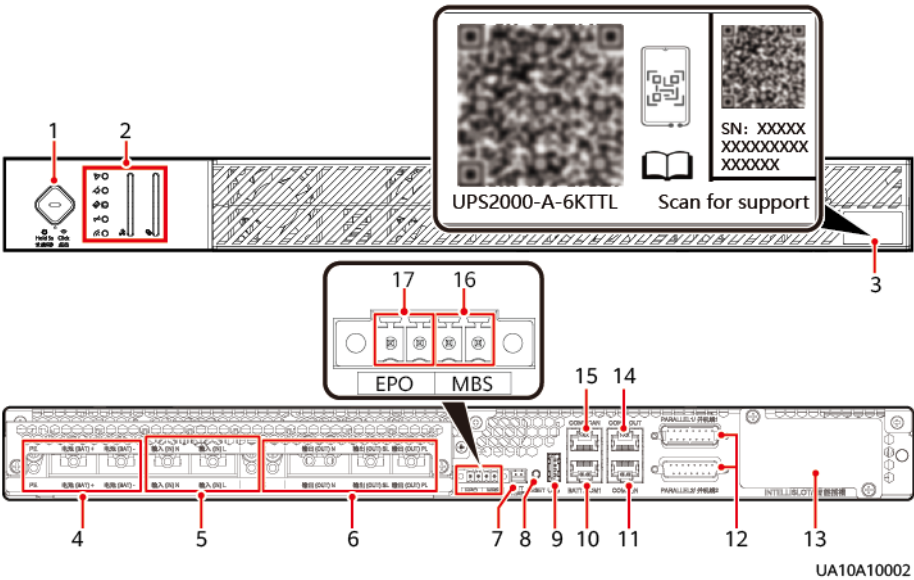
图 4-2 6kVA 外观
